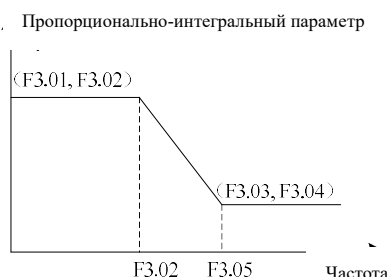
Рис. 6-7 Схема пропорционально-интегральных параметров контура скорости
